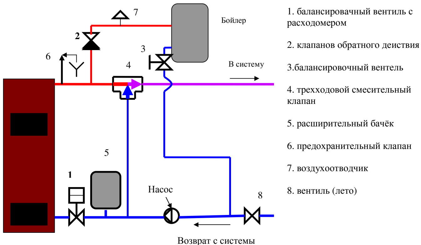
Рис.5 Рекомендуемая схема (бойлер параллельно)
